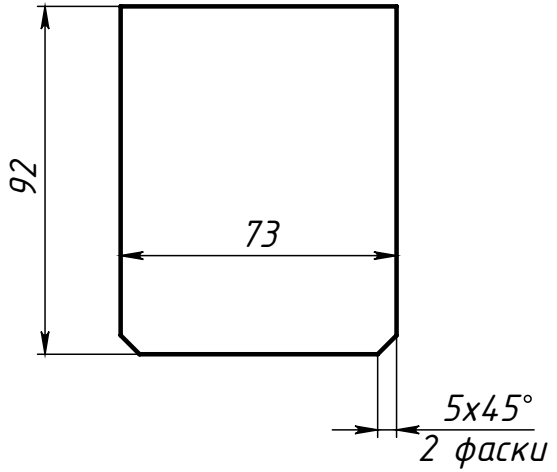
Поз.2 (Ребро)
